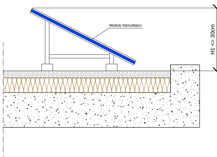
Figura 1 - Caso 1, H \leq 30\text{cm} - Schema esemplificativo di un'installazione idonea alla classificazione dell'impianto fotovoltaico nella categoria "su edifici"
